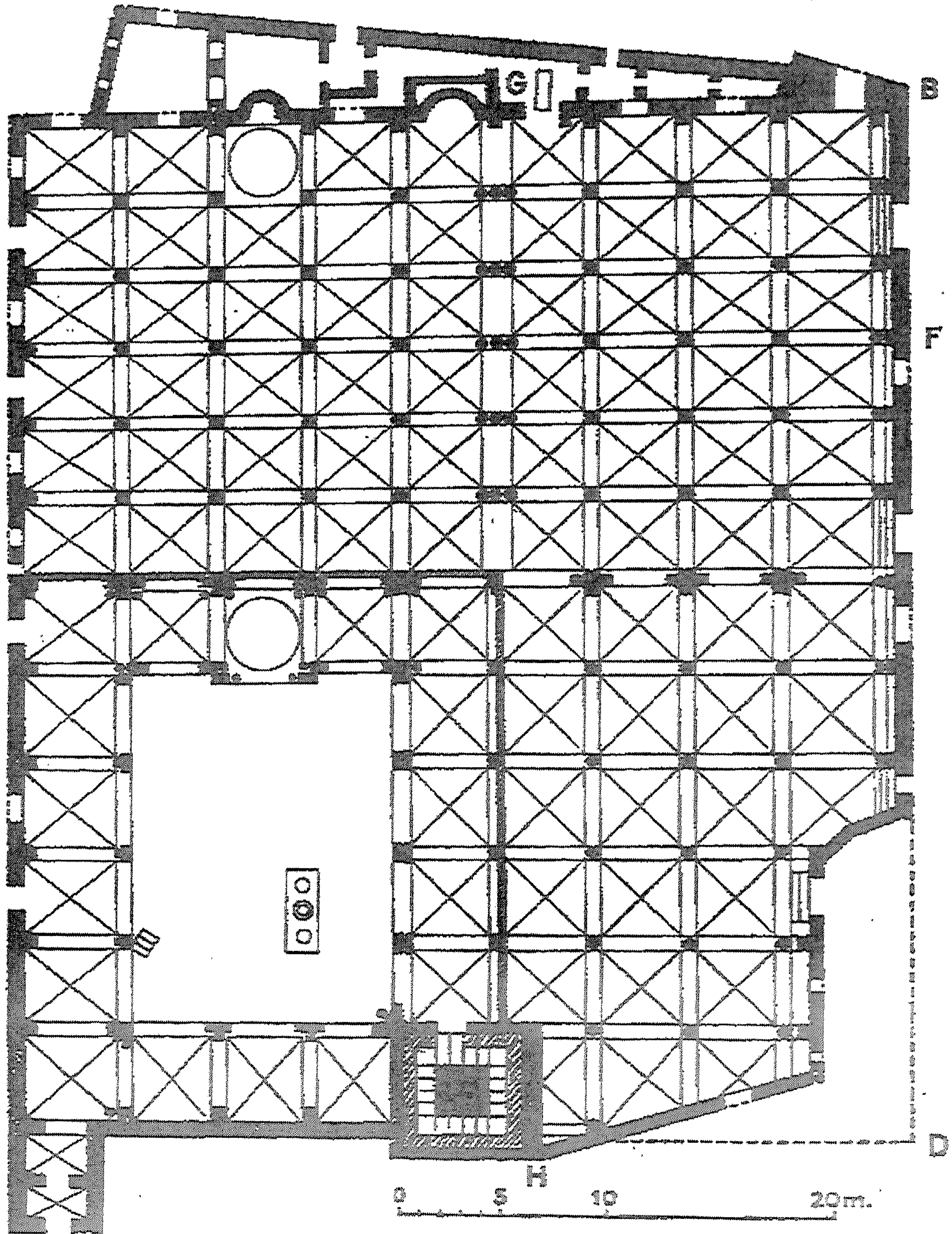
(شكل رقم ٤٢) رسم تخطيطي لجامع صفاقس في العصر العثماني عن جولفان.
